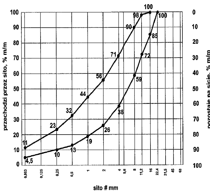
Rys. 3. Krzywe graniczne uziarnienia mieszanki mineralnej 0/16 mm
